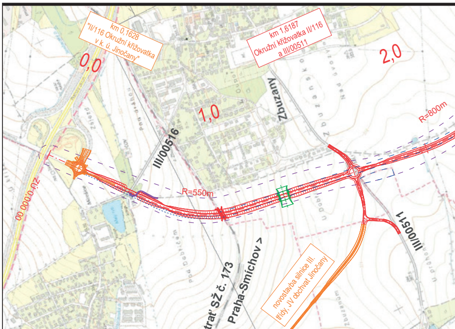
Detail napojení nové propojky na Pražský okruh
